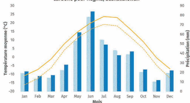
Projections de changement climatique à haute intensité carbone pour Regina, Saskatchewan
